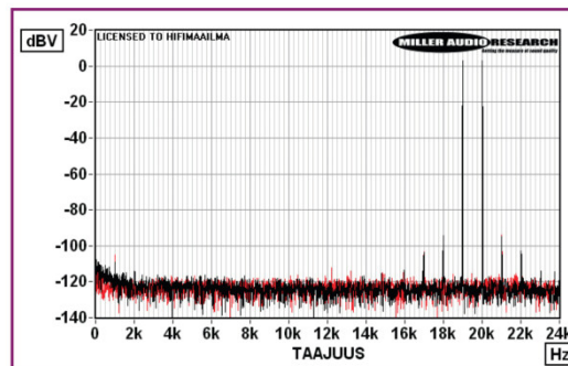
Intermodulaatiospektri 19+20 kilohertsin sinisignaaleilla watin teholla kahdeksaan ohmiin.
