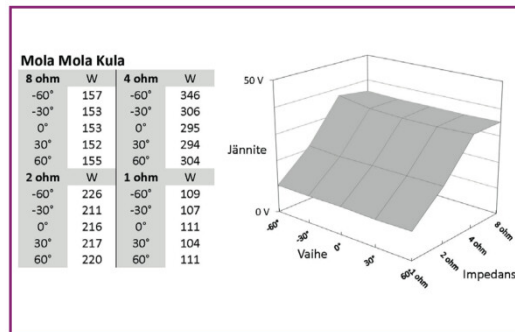
Powercube-tehmittaus eri resistiivisiin ja reaktiivisiin kuormiin.
