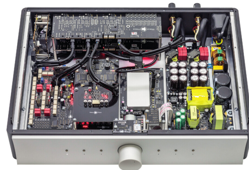
Sitä saat, mistä maksat. Vasemmalla äänivoimakkuussäätimen elektronikkaa, oikealla vahvistinmoduulit virtalähteeseen. Rakenne on lähempänä ammattielektronikkaa kuin hifiä. Esimerkillinen toteutus saa kumartamaan insinöörien suuntaan.
