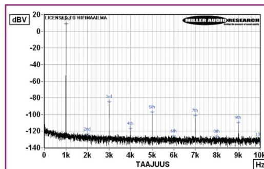
Harmonisen särön spektri yhden kilohertsin sinisignaali-la watin teholla kahdeksaan ohmiin.
