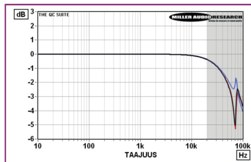
Taajuusvaste kahdeksan ohmin kuormaan (vasen kanava musta, oikea kanava sininen) ja Aurelia Magenta -kaiuttimella (punainen).
